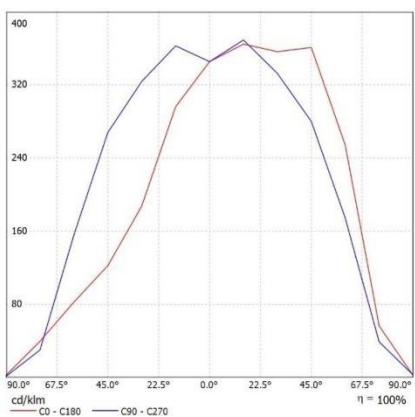
Curba de Iluminare
