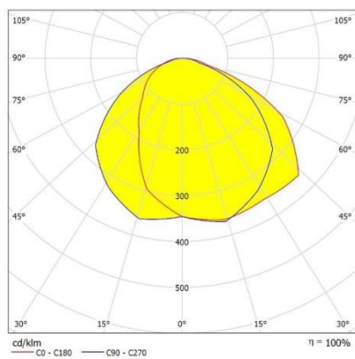
Distributia de Luminanta
